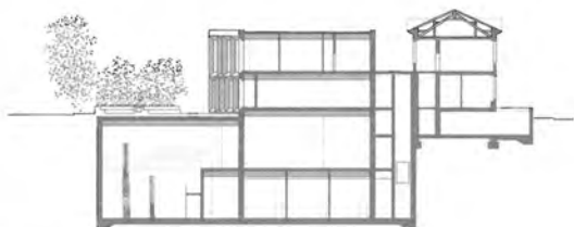
Querschnitt
